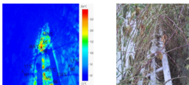
Рисунок 3 – Потери теплоты на выходе теплосети из теплицы № 4: температура снаружи теплоизоляции 59,3 °С, при температуре наружного воздуха -0,4 °С
