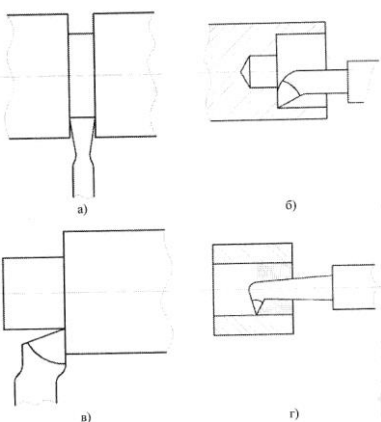
Рисунок 1 - Схемы обработки токарными резцами
